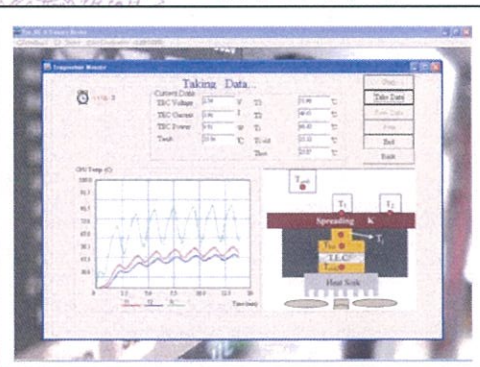
Fig. 8 熱擴散率溫度量測介面圖
